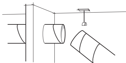
Upphängningsanordningar för ventilationskanaler
