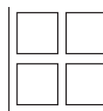
Inbrottsgaller i plåt, t = 4 mm Öppning försett med galler 50x50x10 mm.
